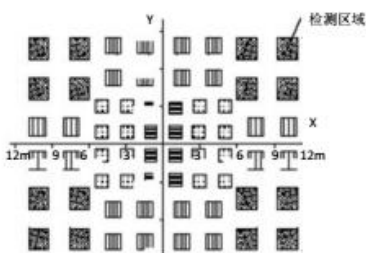
X-Y 截面图
